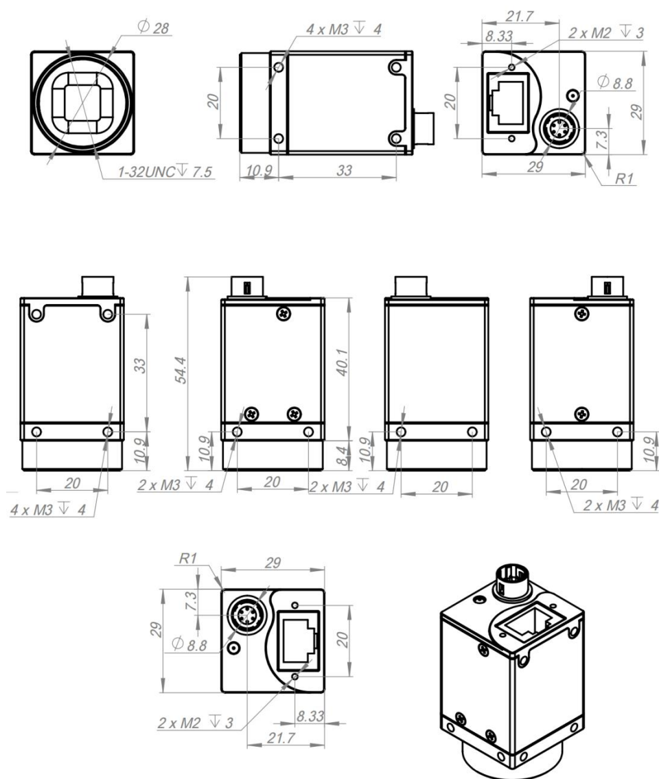
图 5.2 C口产品尺寸图1-V2(单位: mm)
