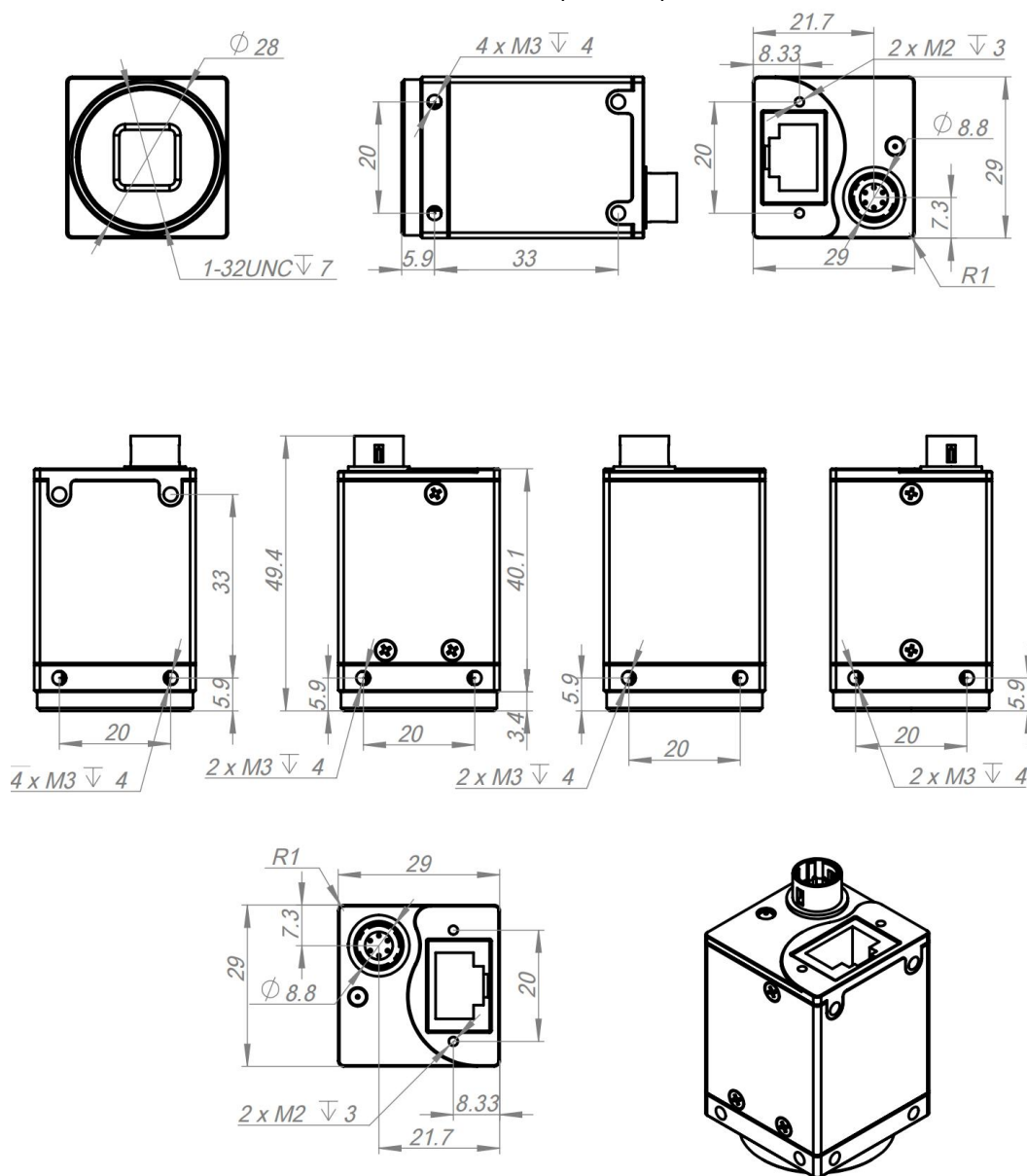
图 5.6 CS口产品尺寸图(单位: mm)
