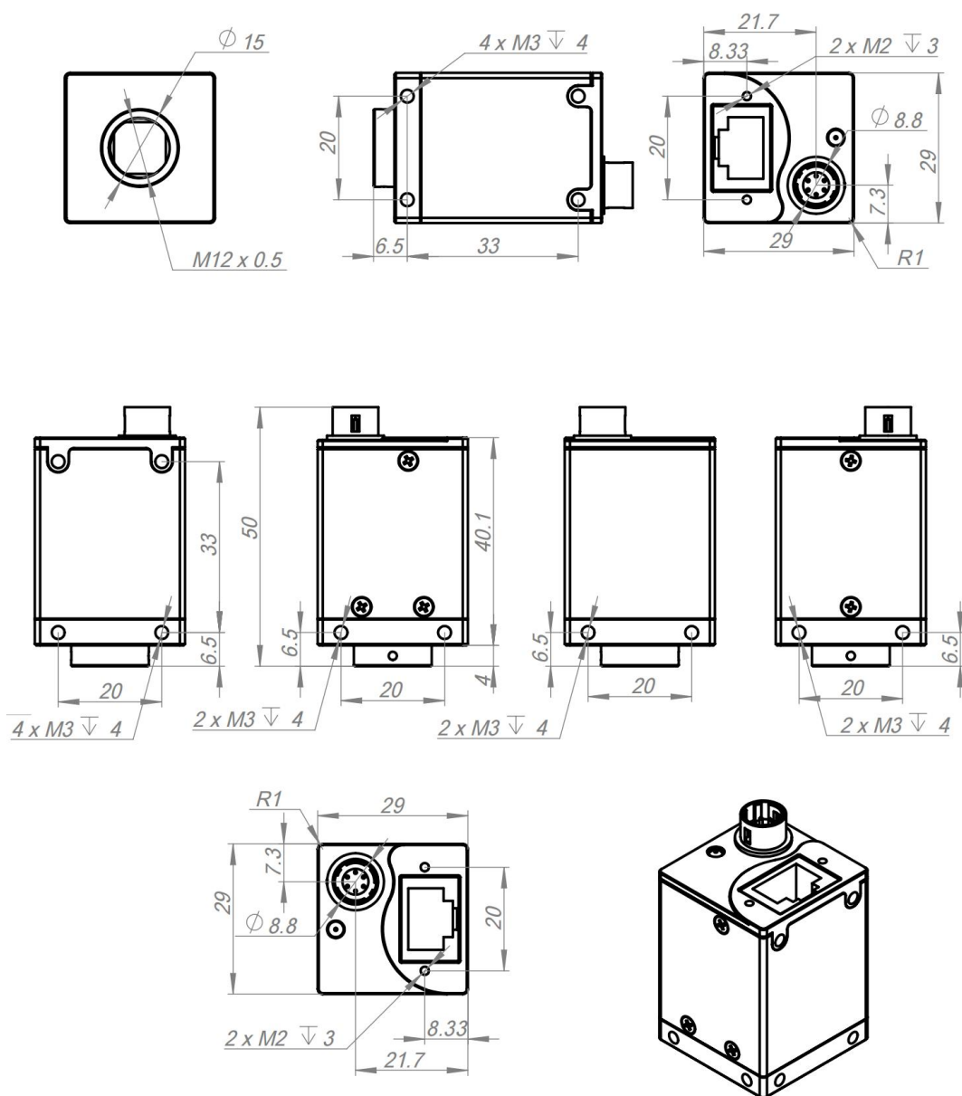
图 5.8 M12产品尺寸图V2(单位: mm)
