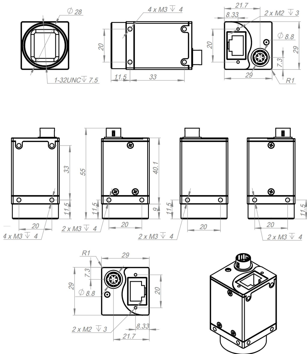
图 5.3 C口产品尺寸图2-V2(单位: mm) (适用型号204, 2000, 800)
