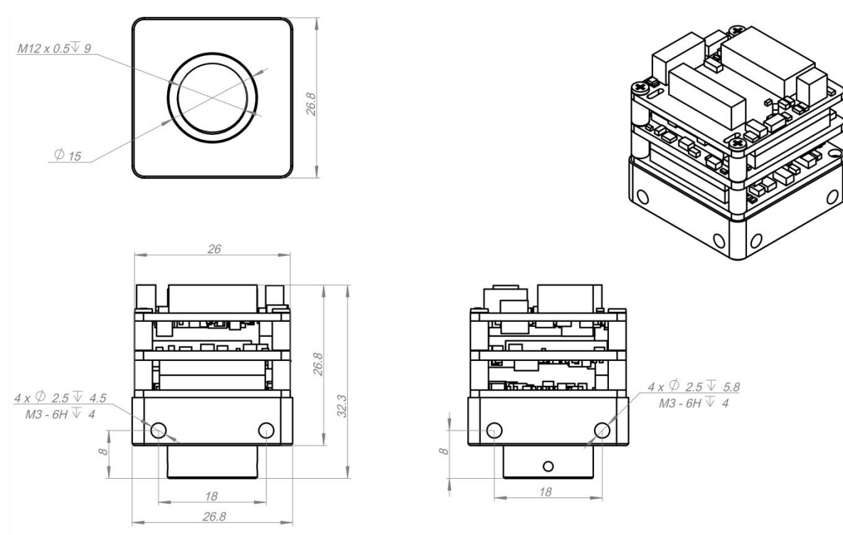
图 5.14 VM模组产品尺寸图(单位: mm)
