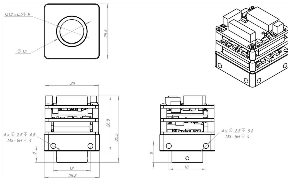
图 5.12 WM模组产品尺寸图(单位: mm)
