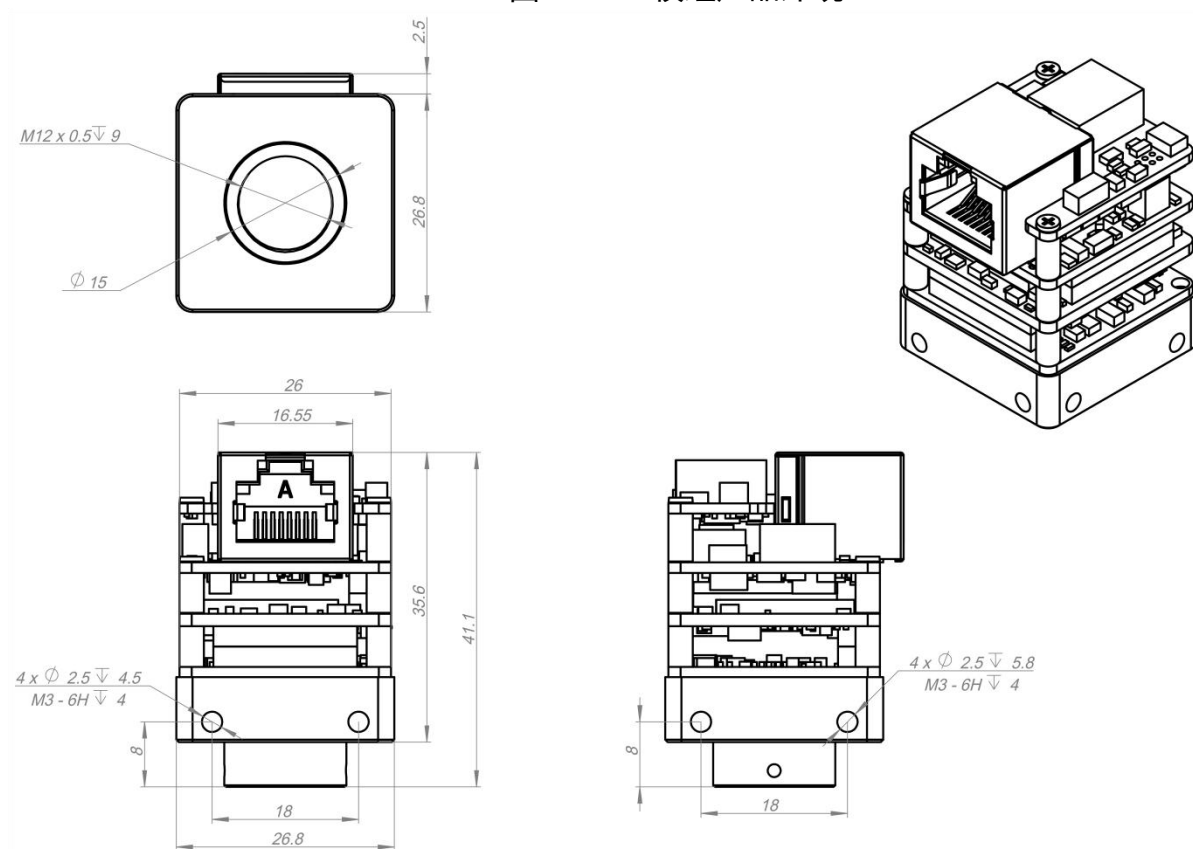
图 5.9 HM模组产品外观
