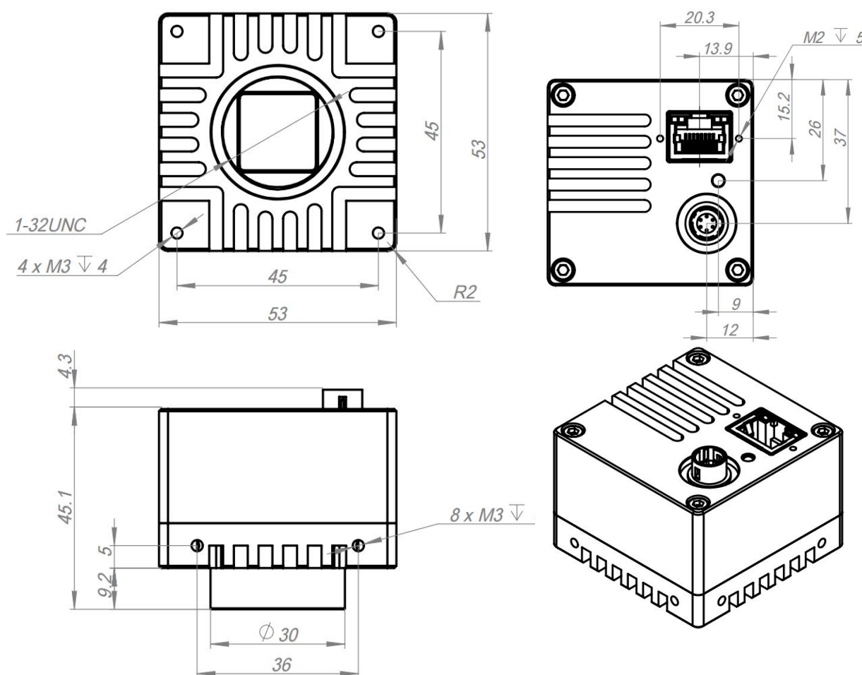
图 5.8 大C口产品尺寸图(单位: mm) (适用型号JHEM508/1608XGM/XGC)
